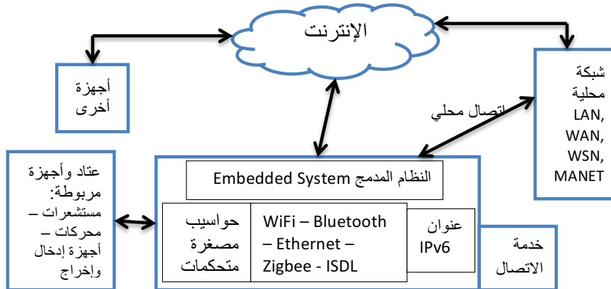
هيكلية مبسطة لنظام انترنت الأشياء (LoT)
